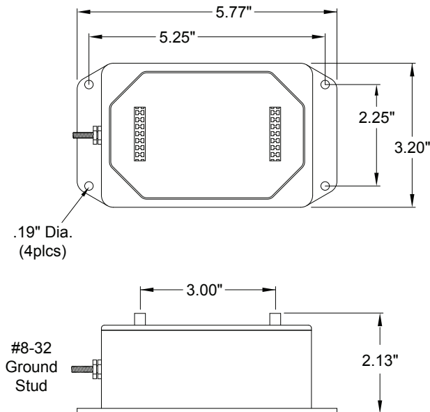
Fig. C - DIMENSIONS
