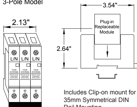
Fig. C - DIMENSIONS
