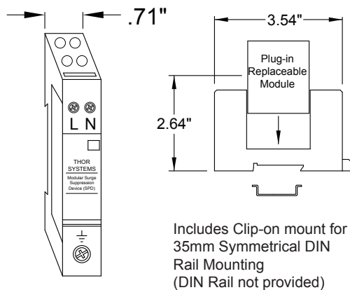
Fig. C - DIMENSIONS
