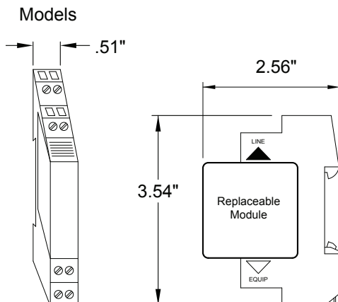
Fig. C - DIMENSIONS
