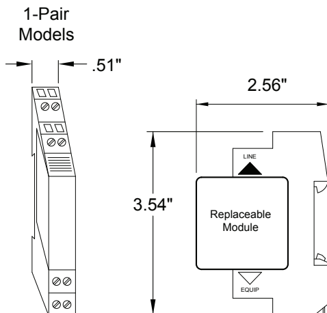
Fig. C - DIMENSIONS
