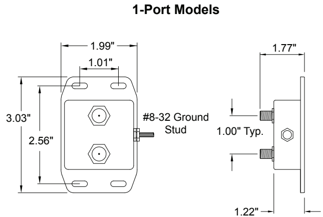
Fig. C - DIMENSIONS
